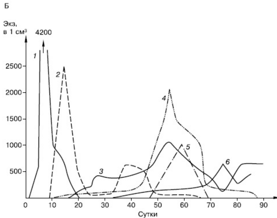
Рис. 154. Смена простейших в сенном настое (по Р. Дажо, 1975): А – общая схема; Б – конкретная серия: 1 – жгутиковые; 2 – инфузории кольноды; 3 – нарамечи; 4 – брюхо- ресничные инфузории; 5 – амебы; 6 – сувойки
