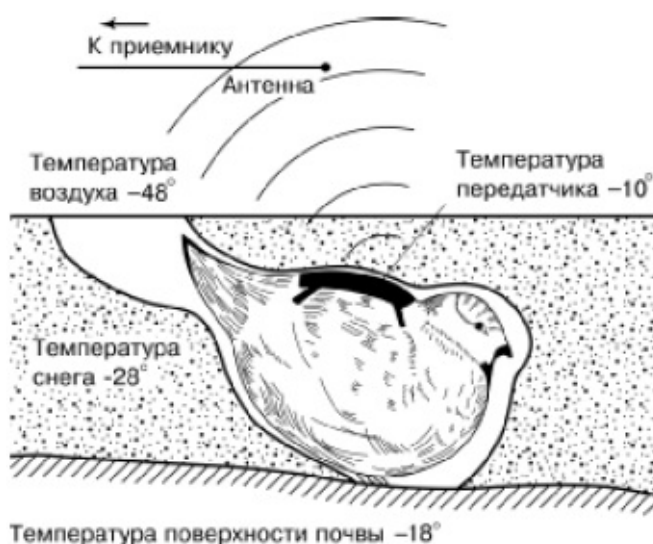
Рис. 48. Схема телеметрического изучения температурного режима ярбчика, находящегося в подснежной лунке (по А. В. Андрееву, А. В.
