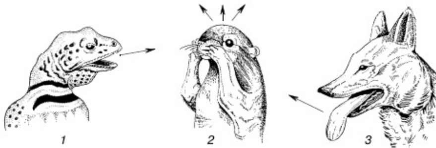
Рис. 17. Испарительная терморегуляция у животных:
