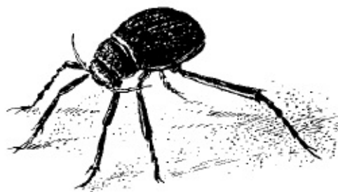
Рис. 111. Жук-чернотелка в пустыне. Одиночный образ жизни
