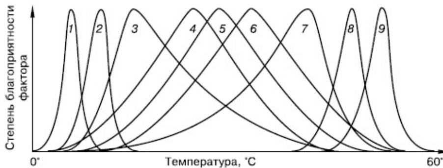
Рис. 2. Положение кривых оптимума на температурной шкале для разных видов:
