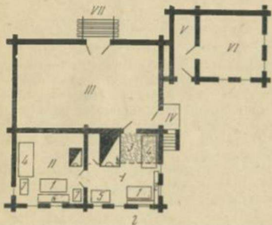
Рис. 4. Дом с боковой зимней избой, соответствующей скотной избе (1), и план того же дома (2) (с. Пучком)
