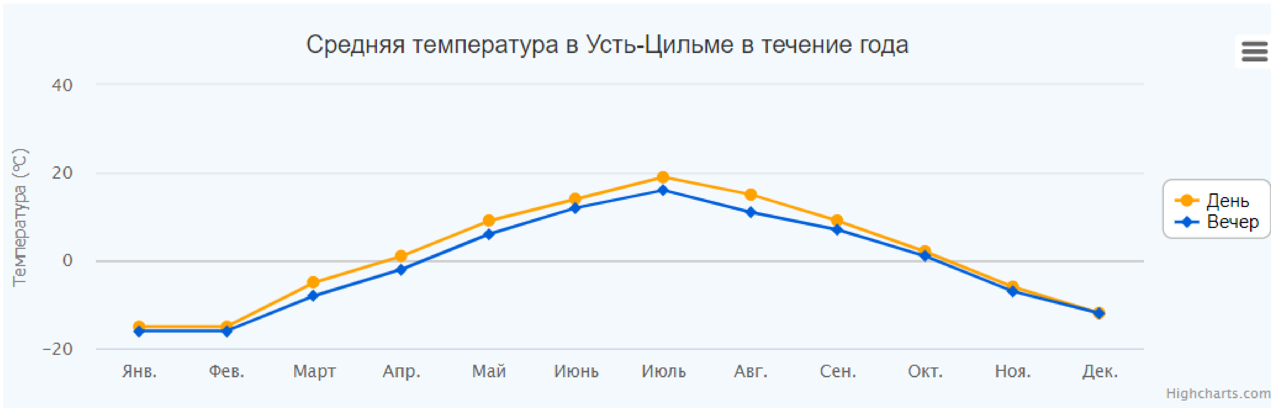
График усредненной дневной и вечерней температуры в Усть-Цильме за историю наших наблюдений
