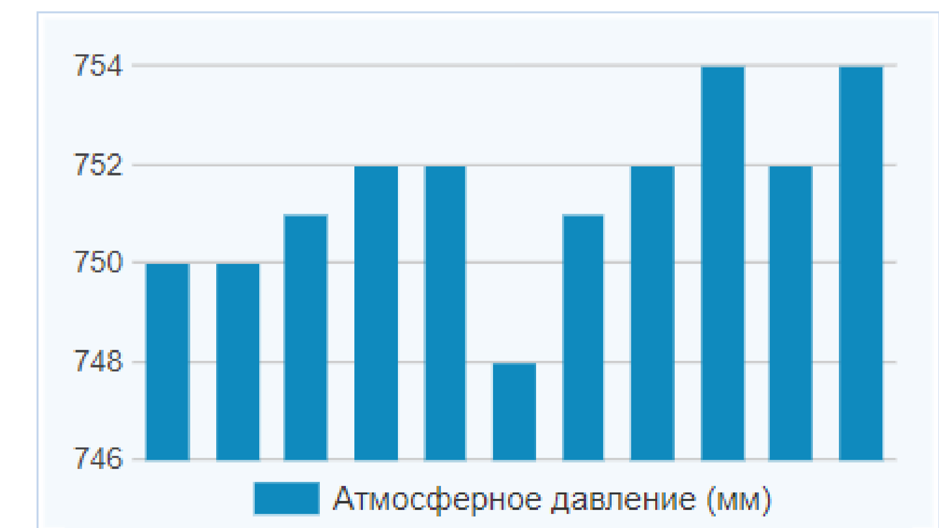
На графике отображено среднее атмосферное давление в Усть-Цильме по годам.
