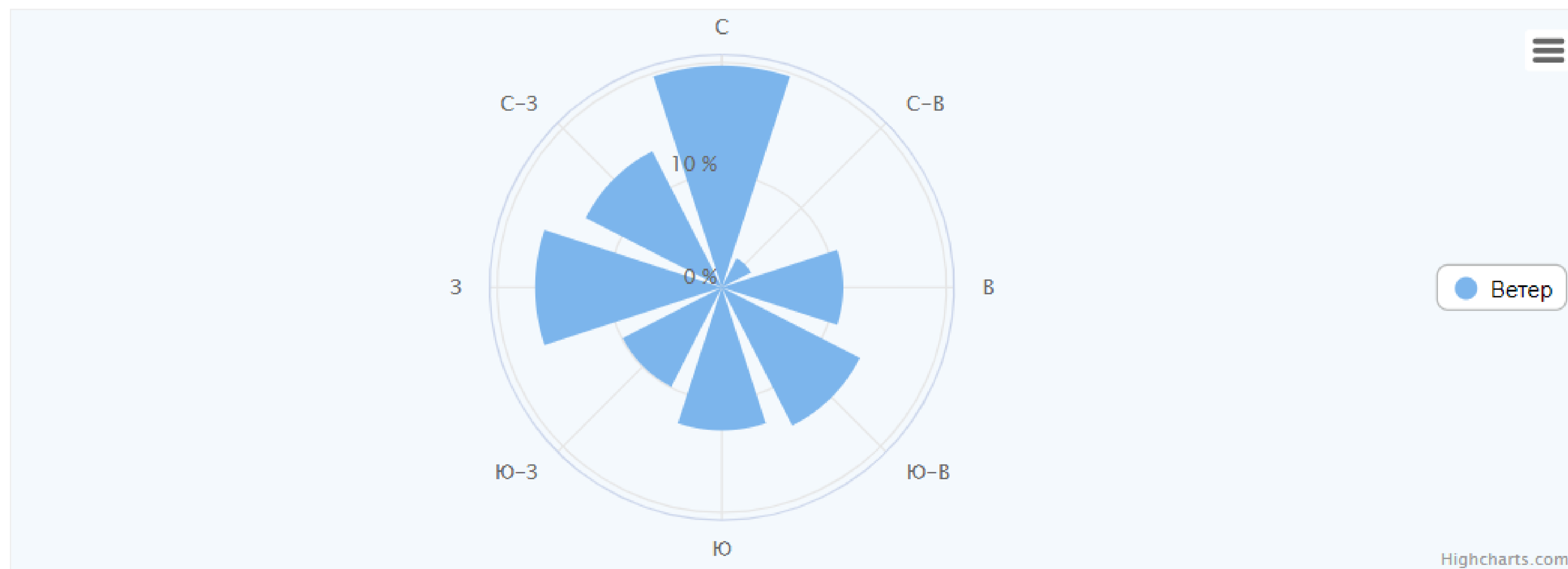
График ветра (направление - откуда дует ветер) в Усть-Цильме, с усредненными значениями согласно нашим данным.
